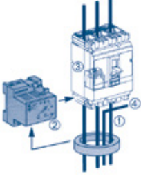
① Toroid ② Vigiex röle ③ MX bobini ④ Nötr
