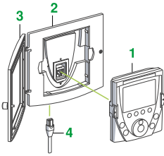
ATV71 uzaktan bağlantı kiti
