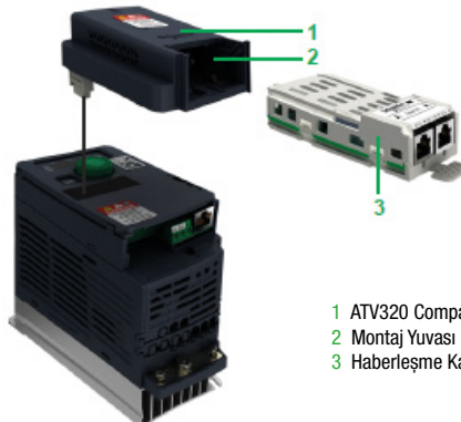
Haberleşme Kartı Montaj Örneği
